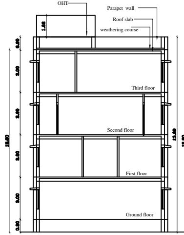
SECTION X, Y
